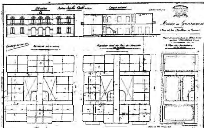
Planta arquitectónica, fachada y sección del Palacio de Gobierno provincia Bocas del Toro (1907)
