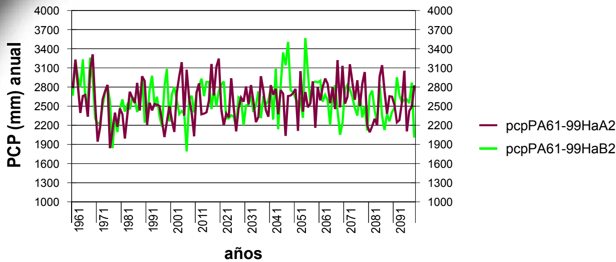
PCP anual Panama 1961-2099 HadCM3 A2 vs B2
