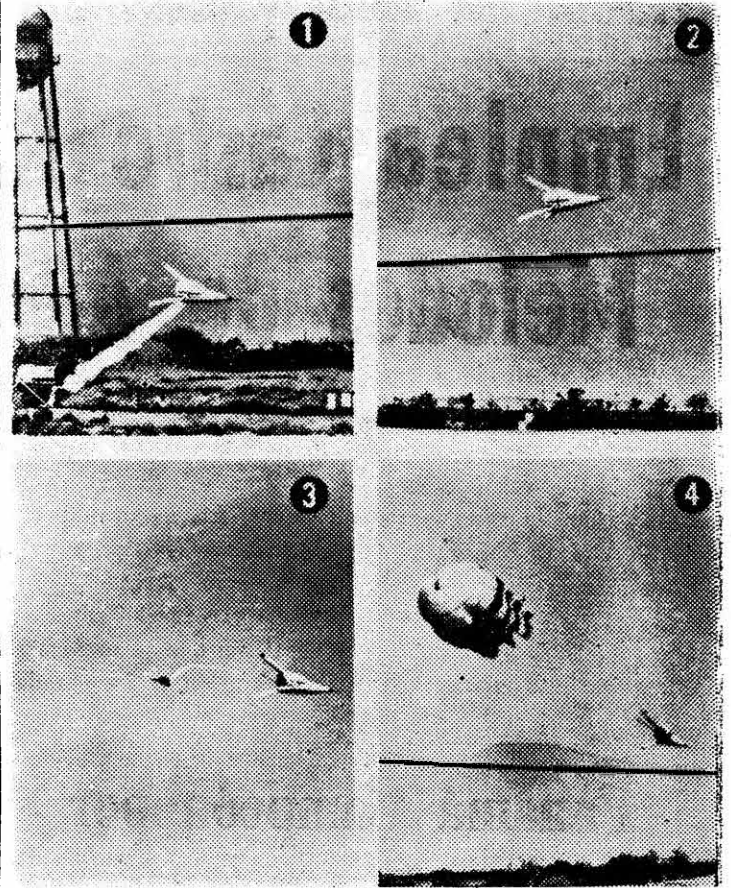
UN PROTOTIPO DE CAPSULA DE ESCAPE PARA AVIONES, desarrollado por la Compañía Lockheed-California, diseñado para proteger a los pilotos que tuvieran que abandonar futuros aviones de 2.500 m.p.h. en altitudes de 100.000 pies donde el aire es delgado y la temperatura congelante, pasó con todo éxito las pruebas a que fue sometida en la Base Aérea de Edwards, Calif. Las fotos en secuencias muestran (1) separación de la cápsula no tripulada, pero dotada de instrumentos, del vehículo que simula el fuselaje, después que toda la unidad corrió por la pista de alta velocidad; (2) la cápsula de tres alas con 2.400 libras de presión (incluido un "piloto" de 160 libras dentro) en vuelo libre; (3) lanzamiento del paracaídas de 5 pies de diámetro; y (4) apertura del paracaídas de recuperación de 72 pies de diámetro que permite un aterrizaje seguro de la cápsula a unas 19 millas por hora.
